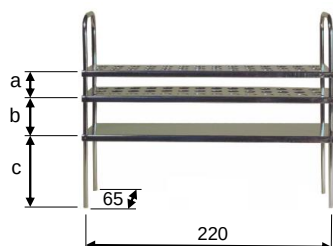
Reagenzglasgestell für Wasserbäder MWB 5 - MWB 40
